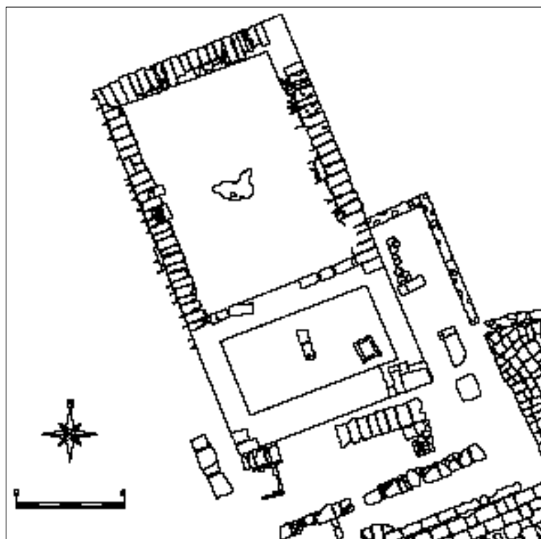
Fig. 20 - Nora. Pianta del Tempio del foro (rilievo A. Faggini, restituzione I. Cerato).
