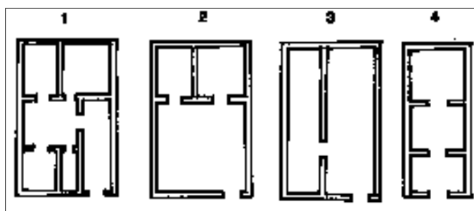
Fig. 77 - Tharros. Tipologie di abitazioni (da FALCHI 1991).
