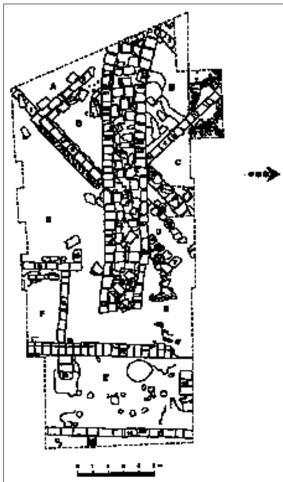
Fig. 12 - Porto Torres. Pianta del tratto murario realizzato in età altomedievale sulle strutture dell' horreum rinvenute presso la Banca Nazionale del Lavoro (da SPANU 1998).
