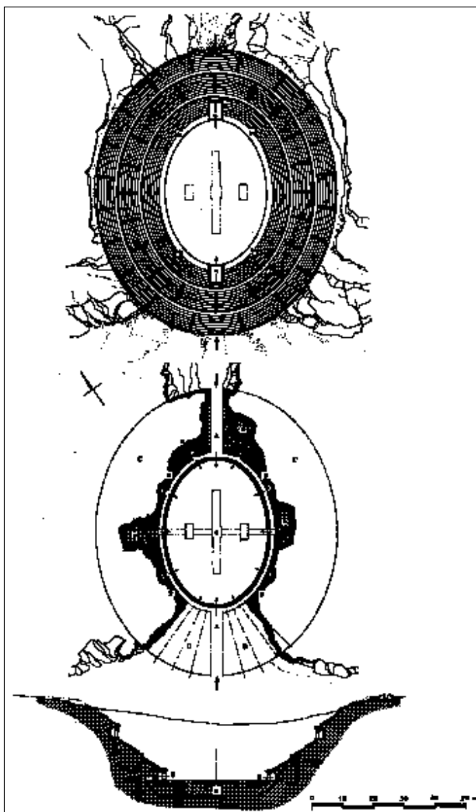
Fig. 40 - Cagliari. Ricostruzione planimetrica, pianta delle strutture ipogee e sezione Nord-Ovest/Sud-Est dell'anfiteatro (da GOLVIN 1988).
