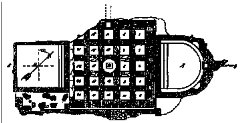
Fig. 64 - Cagliari. Pianta del frigidarium delle Terme suburbane di Bonaria (da TARAMELLI 1909).
