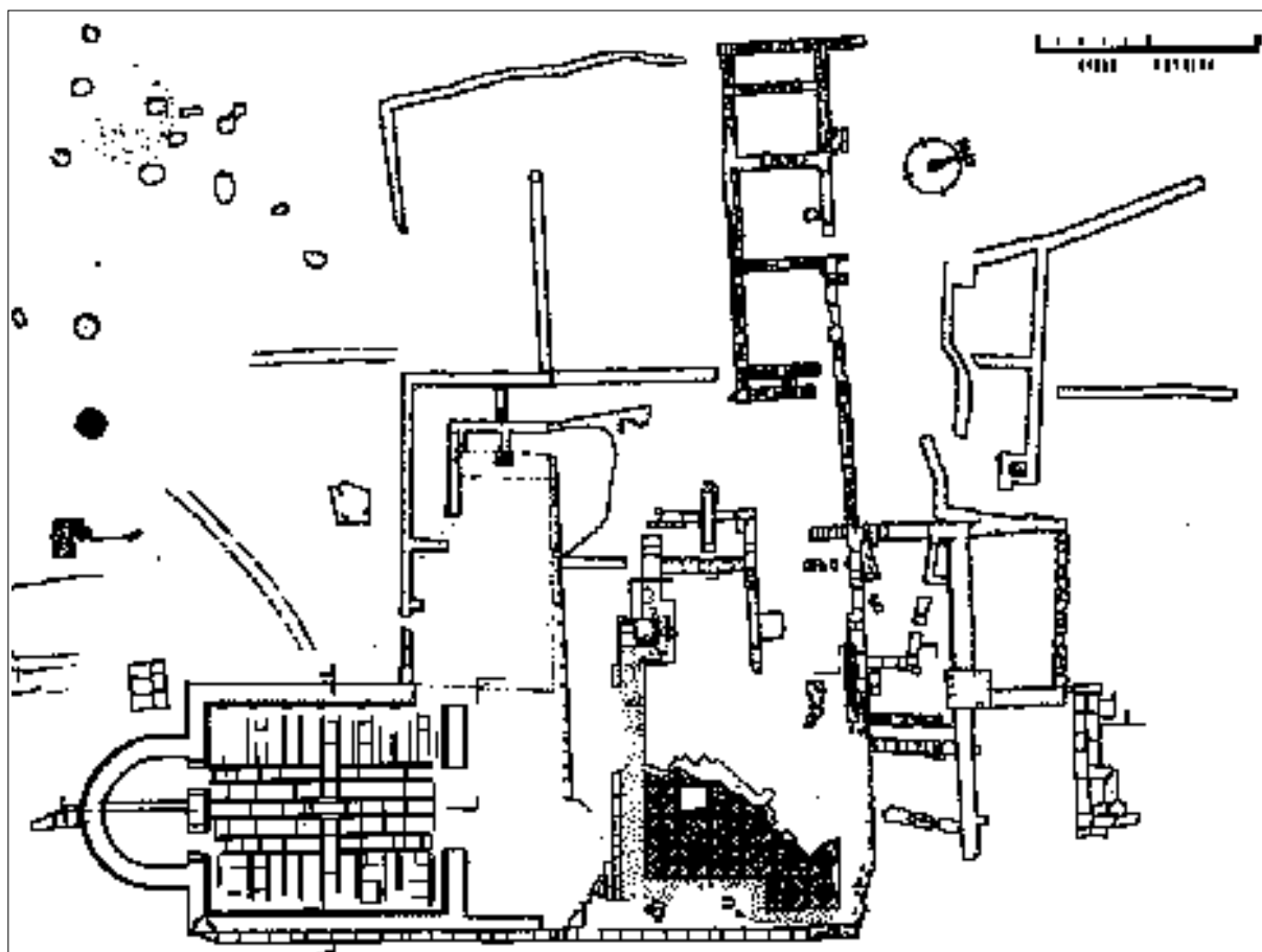
Fig. 26 - Nora. Pianta del «Tempio di Esculapio» (da PESCE 1972 2 ).
