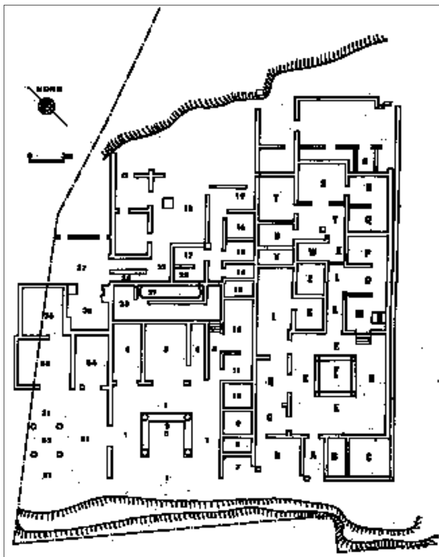
Fig. 80 - Cagliari. Pianta della «Villa di Tigellio»: da Sud-Est verso Nord-Ovest, la «Casa del Tablino dipinto», la «Casa degli Stucchi» e la terza abitazione solo parzialmente scavata (da ANGIO-LILLO 1987).
