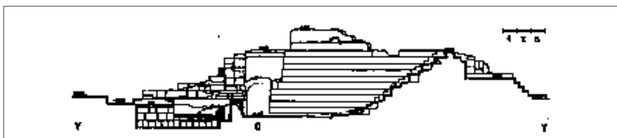
Fig. 37 - Nora. Sezione Sud-Est/Nord-Ovest del teatro (da AMUCANO 1994).
