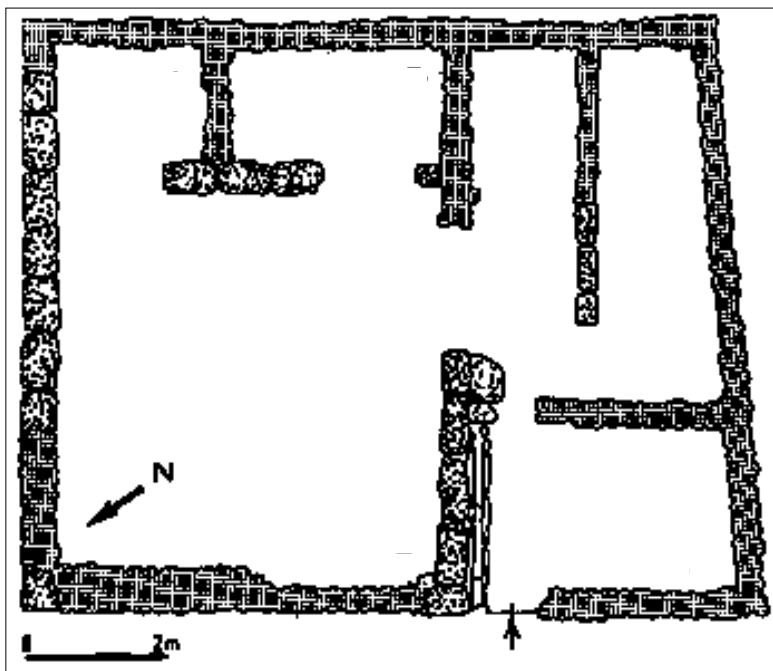
Fig. 78 - Monte Sirai. Pianta della «Casa Fantar» (da BARTOLONI, BONDÌ, MARRAS 1992).
